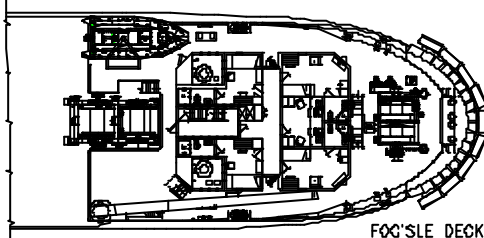
FOG'SLE DECK
